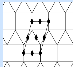
(d) Elongated triangular tiling
