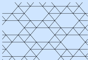
(d) Reverse snub hexagonal tiling t_{\mathcal{T}} = 6
