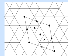
(d) Snub hexagonal tiling
